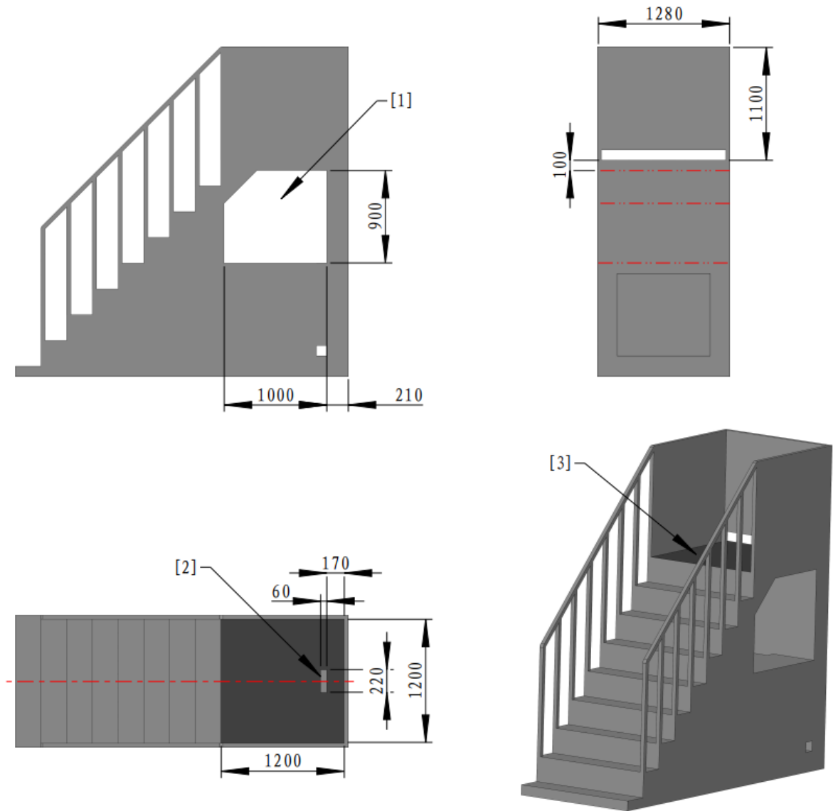
[1] 雷达运算端放置平台 [2] 传感器数据线槽孔 [3] 铁质板材
