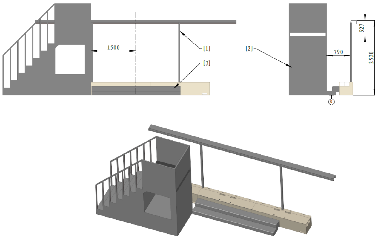
[1] 电动门 [2] 雷达基座 [3] 出入口台阶
